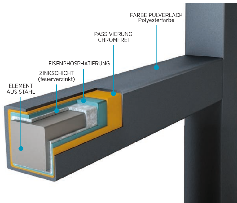
Querschnitt durch das Sicherungselement im System DUPLEX .
